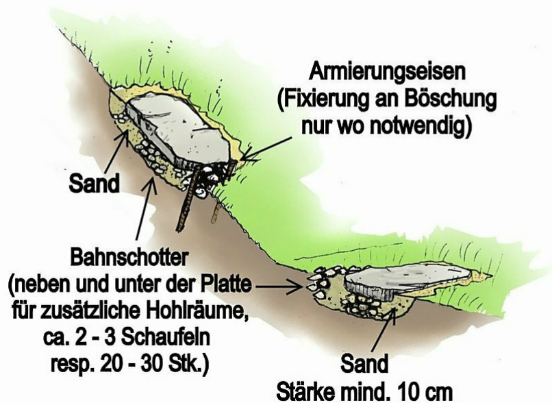
Abb. 2: Steinplatten, links eingebettet, rechts auf Boden aufgelegt
